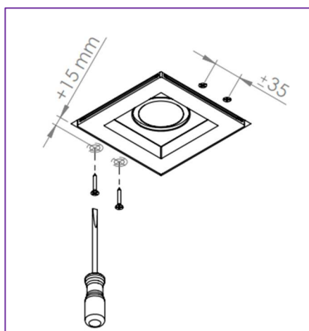
Fig. 4: Vast schroeven gipsarmatuur in het plafond
