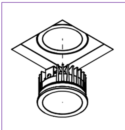
Fig. 8: Plaats led-spot of aanwezigheidsmelder in het gipsarmatuur.
