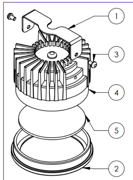
Fig. 7: Samenstelling van de led-spot of aanwezigheidsmelder met de Lumunex montage onderdelen.
