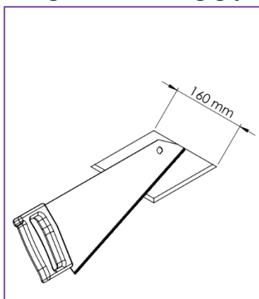
Fig. 1: Gat zagen 160x160 mm
