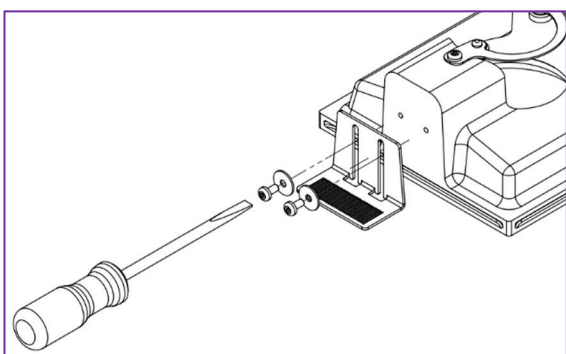
Fig. 3: Montagehoeken bevestigen op de juiste hoogte.
