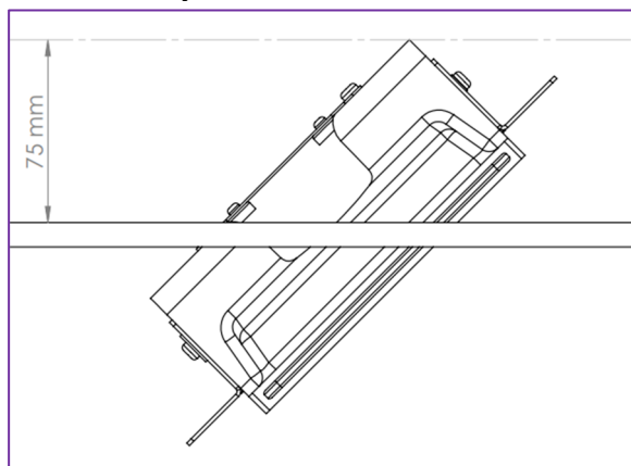
Fig. 2: Gipsarmatuur schuin door het gat steken. Minimale montagehoogte 75mm
