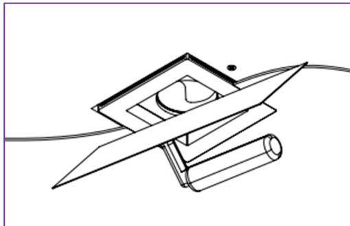
Fig. 6: Stukadoren van het plafond en de gipsarmaturen.
