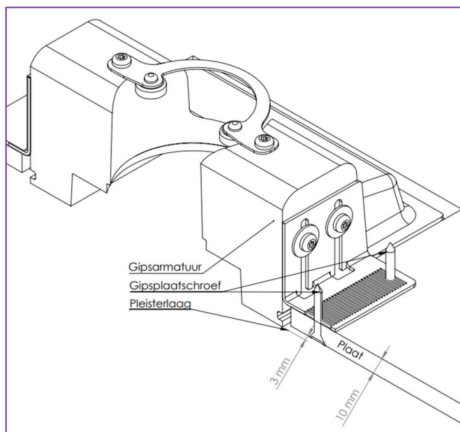
Fig. 5: Voorbeeld maatvoering voor de montage van het gipsarmatuur (let op! doorsnede)
